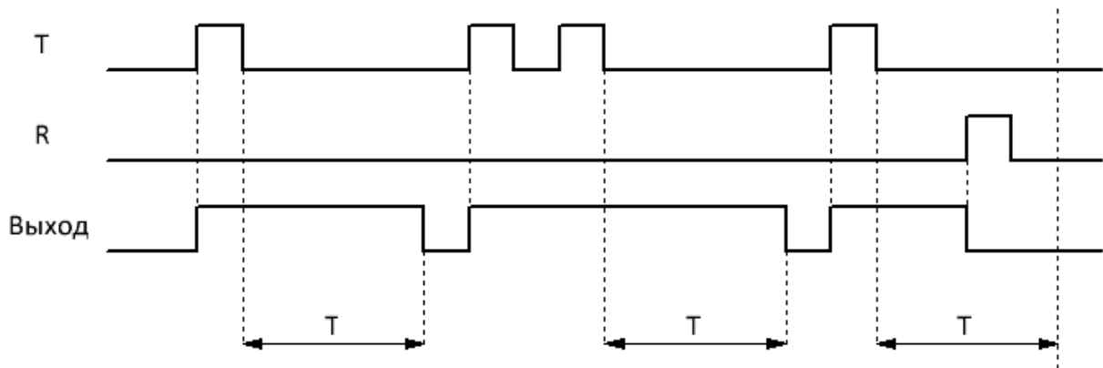
Временная диаграмма
