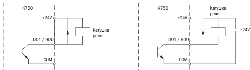
Рисунок 3.2.12 – Схема подключения цифровых выходов
